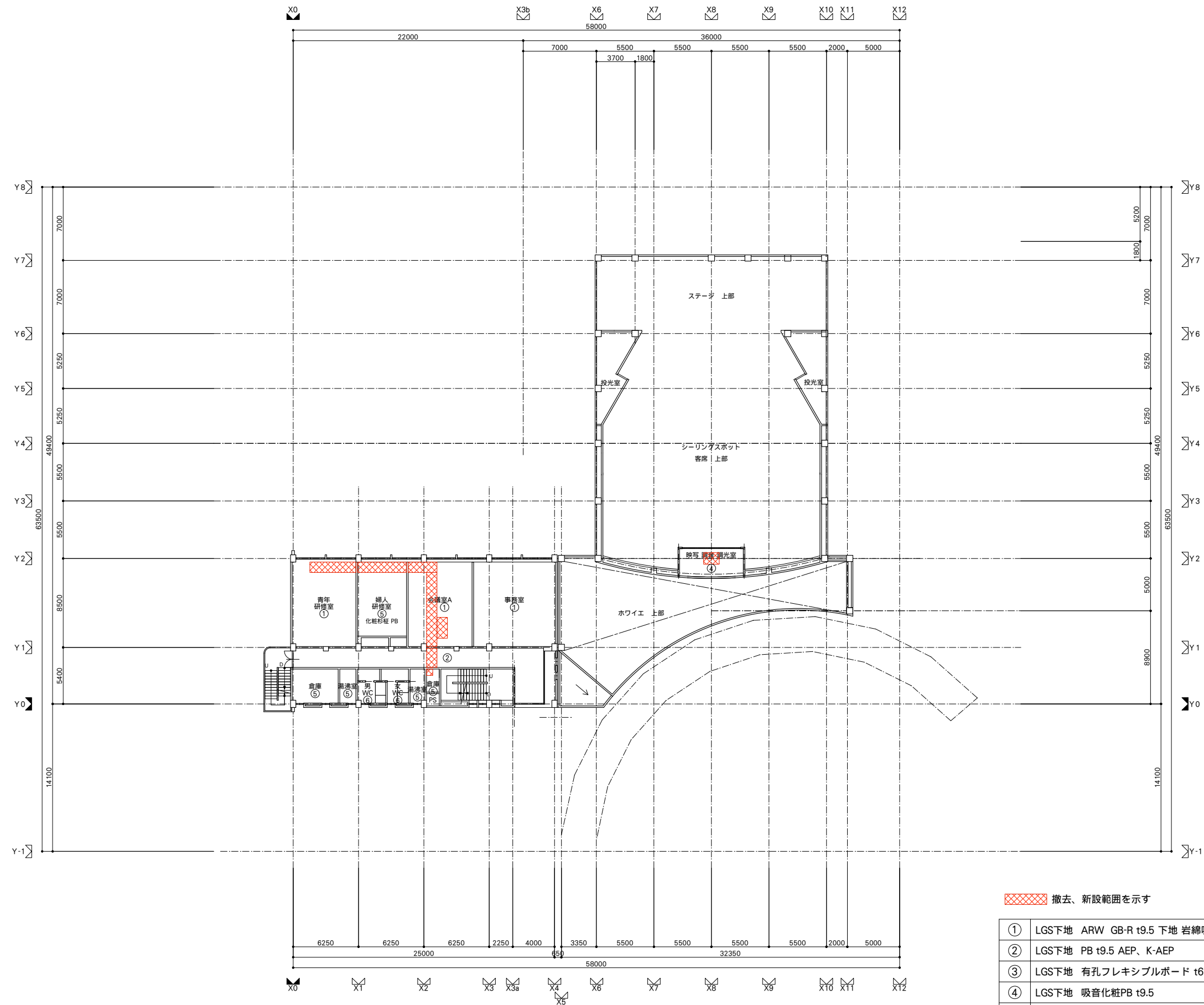
2階天井伏図
